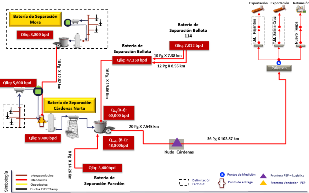
Diagrama de Punto de Medición para la Compraventa Campo Cárdenas - Mora Situación futura
